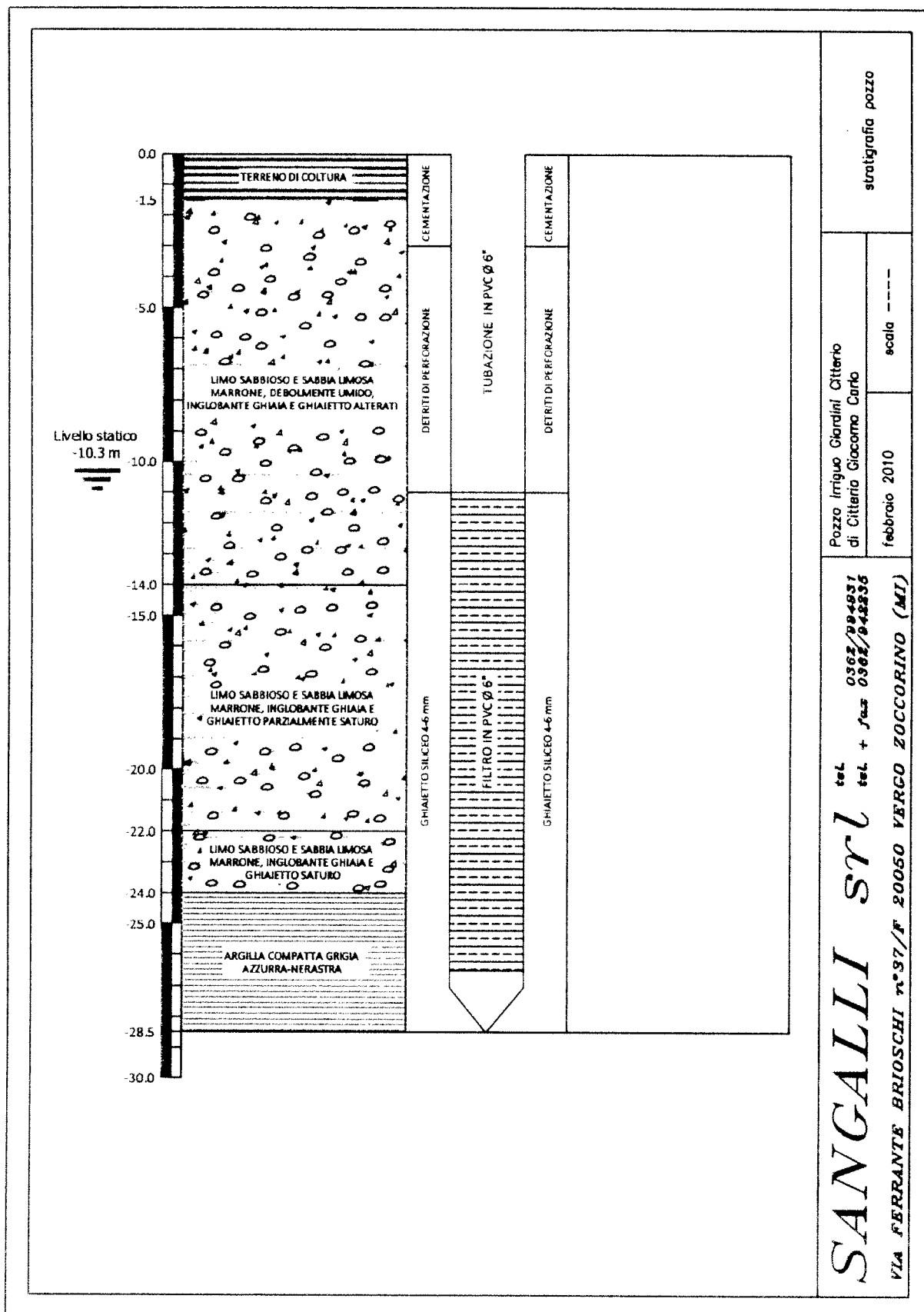
Figura 16 – stratigrafia pozzo Giardini Citterio di Citterio Giacomo Carlo
